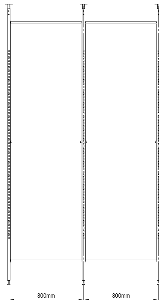
■ 800 mm udaljenosti između centralnih linija vertikalni šina. Opcija bez drvene obloge.
