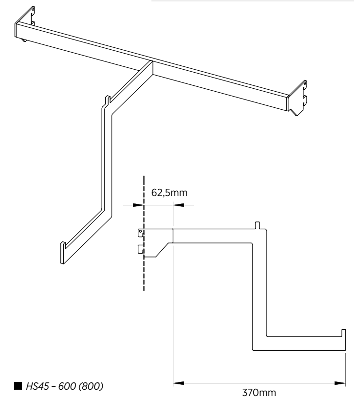
Nosač 45 = HS45
