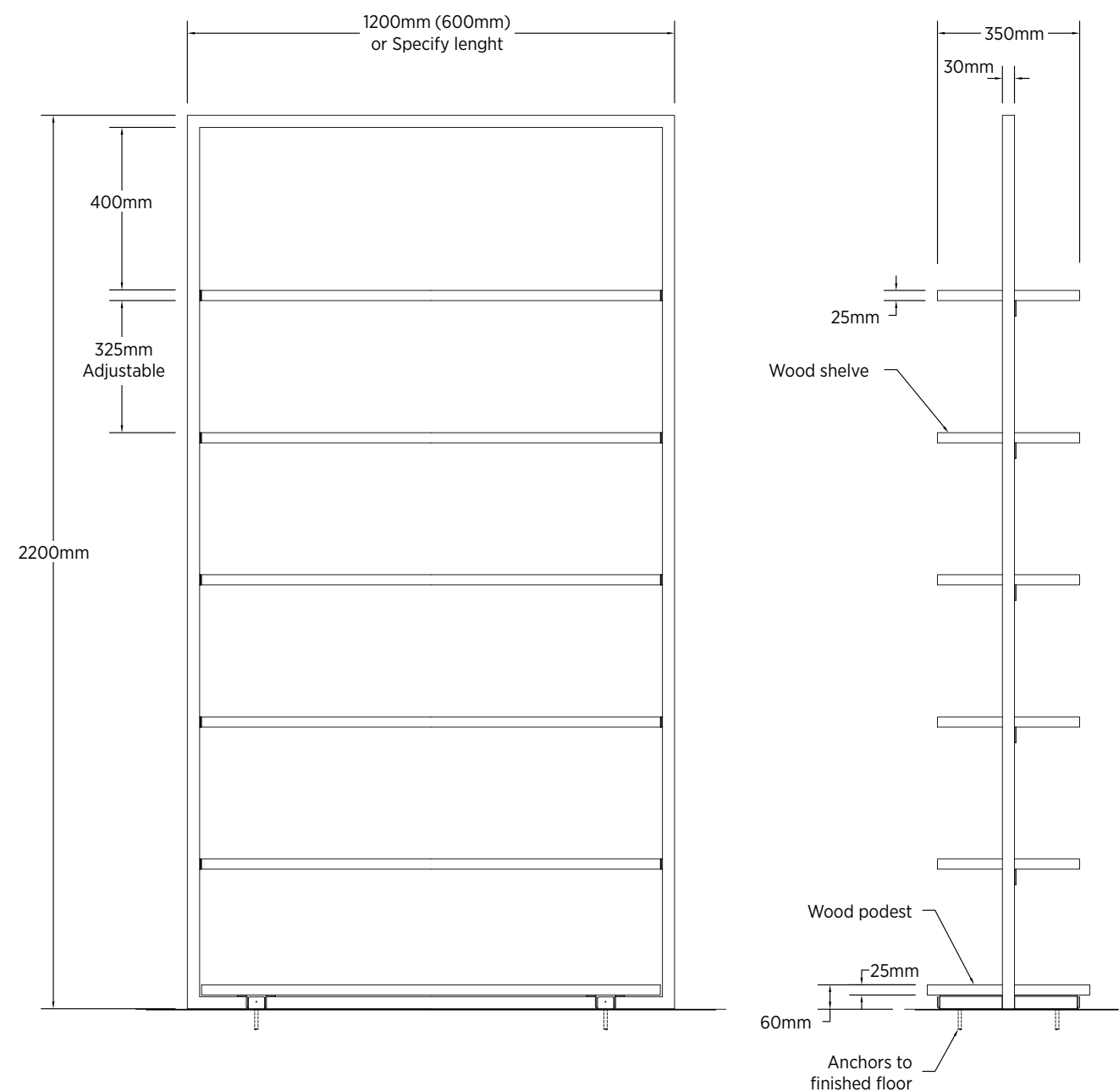
■ FPS – Opcija 3, WS
