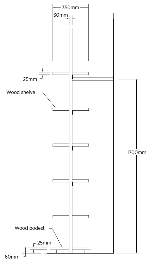
■ FWS - Opcija 3, WS
